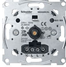
Dimmer mekanizması
